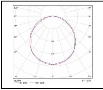
TYTAN 2 LED
