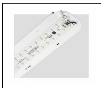
TYTAN MULTI LED 1150mm 2500-4300lm 840 - světelný modul (358937)
