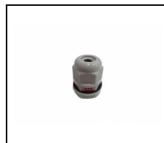
Drüse Entlüftung verschiedene grau M20*1.5 IP68 (16000507)
