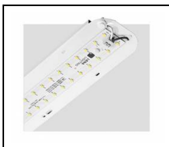
TYTAN LED 1450mm 6500/10300lm 830 - moduł świetlny (907302)
